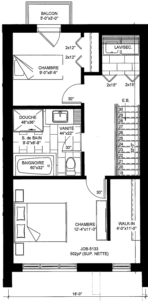
2e ÉTAGE
