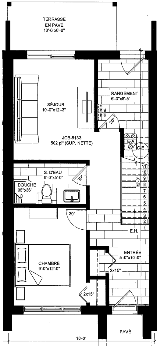
REZ-DE-CHAUSSÉE
