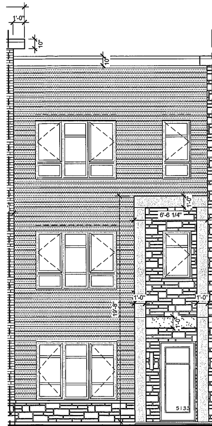
ÉLÉVATION
