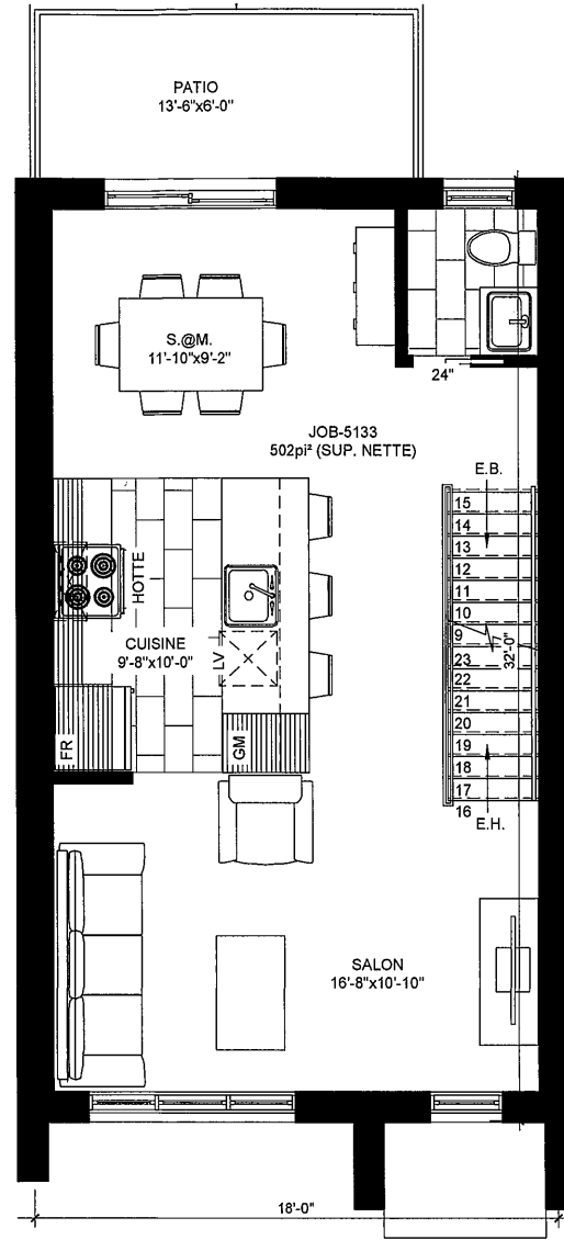
ÉTAGE
