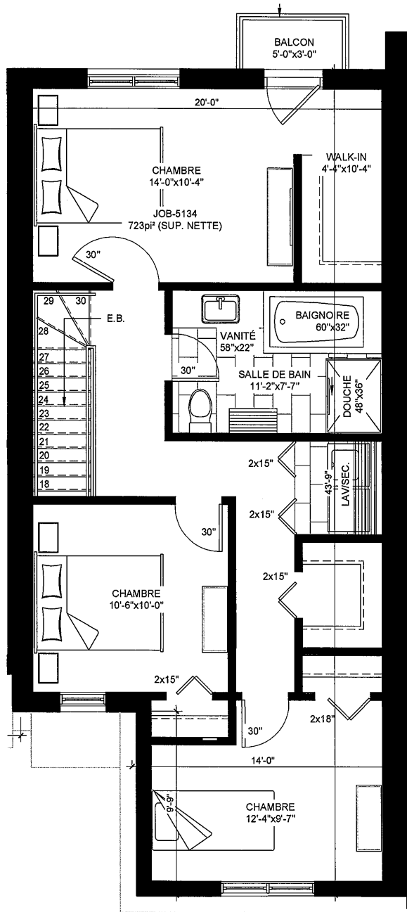
2e ÉTAGE
