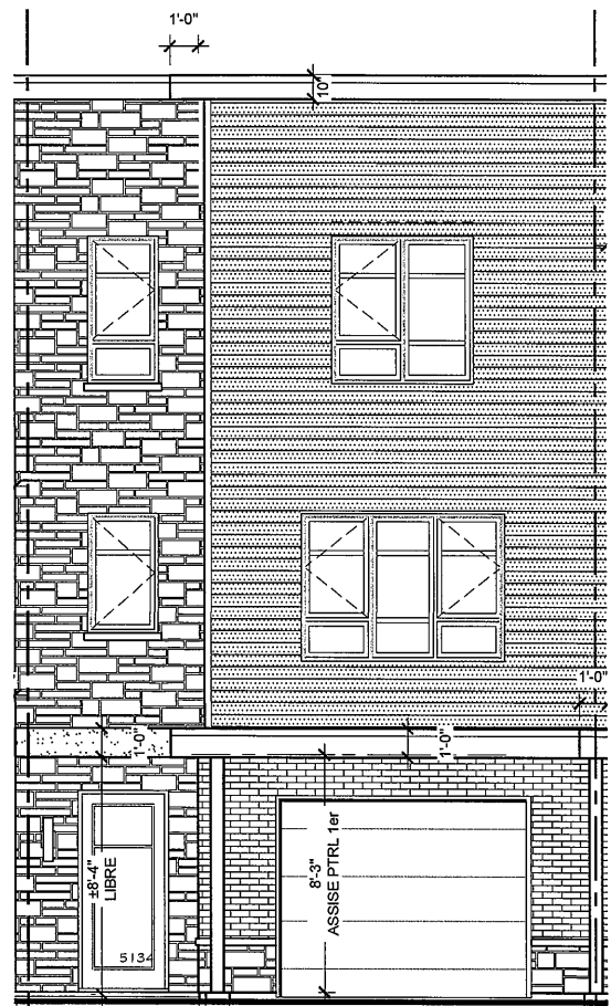
ÉLÉVATION
