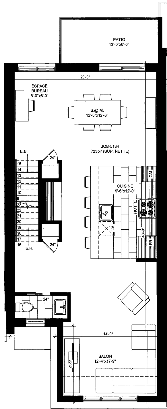
ÉTAGE
