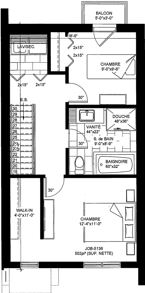
2e ÉTAGE
