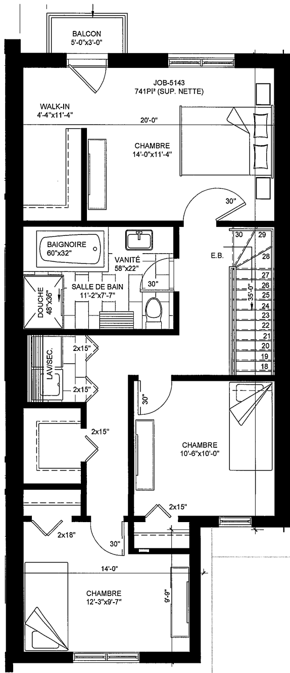
2e ÉTAGE
