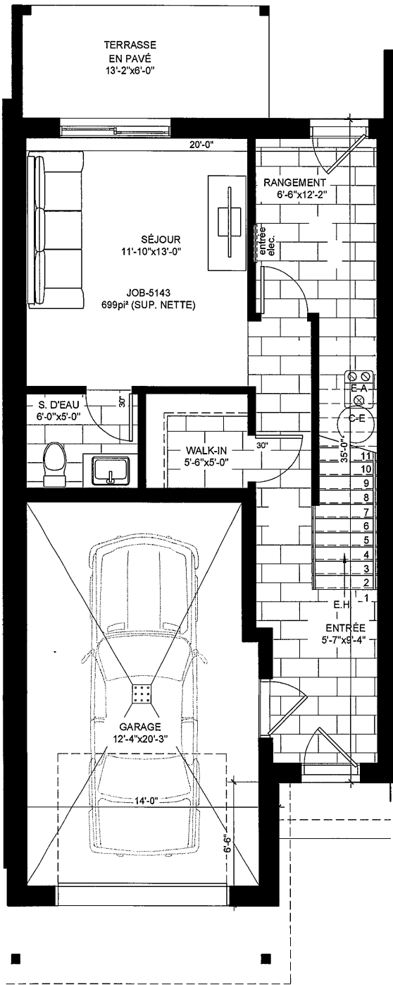
REZ-DE-CHAUSSÉE
