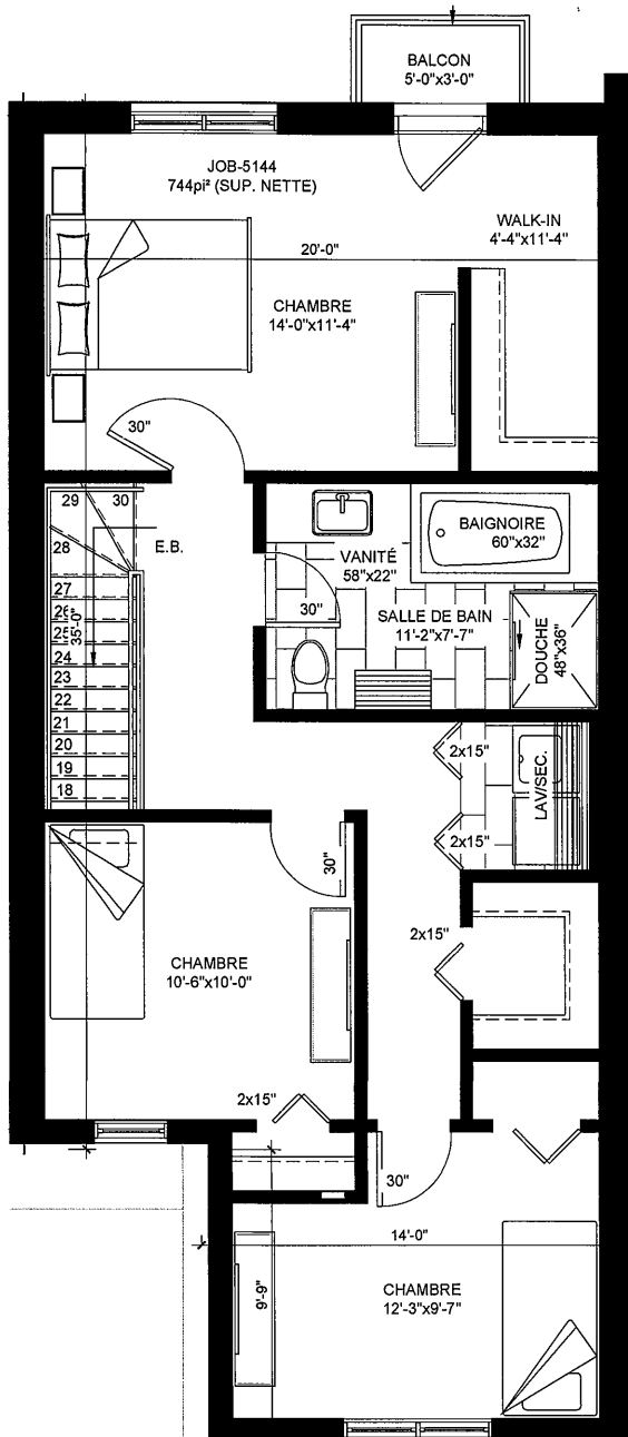
2e ÉTAGE
