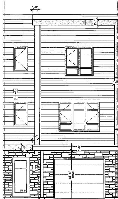
ÉLÉVATION
