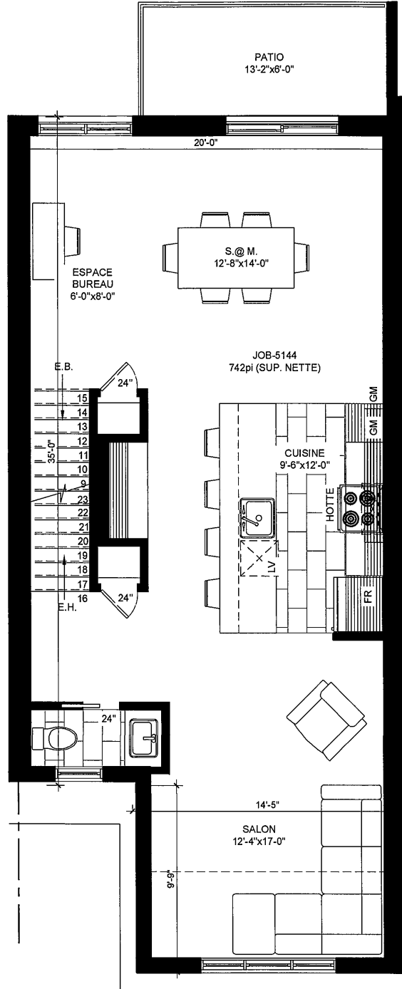
ÉTAGE
